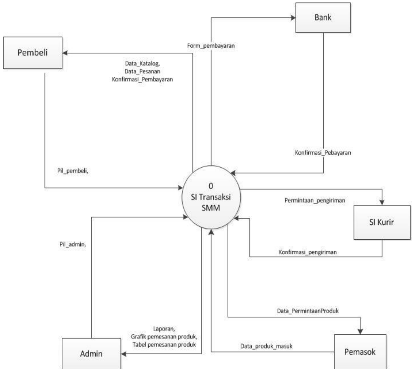
Gambar 2. Diagram konteks SI Transaksi SMM
