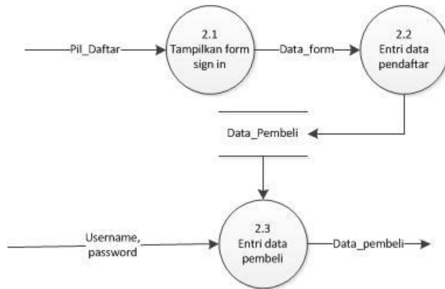
Gambar 4. Diagram Level 2 Proses pendaftaran
