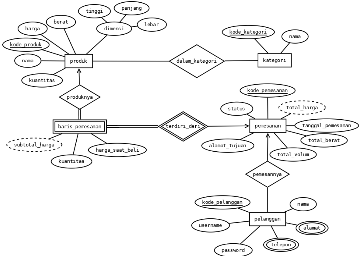
Gambar 10. Diagram ER
