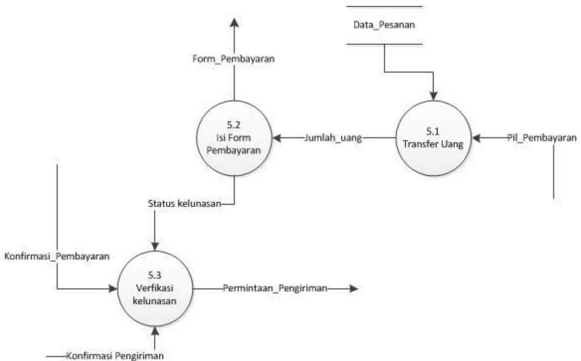
Gambar 7. Diagram Level 2 Proses Pembayaran
