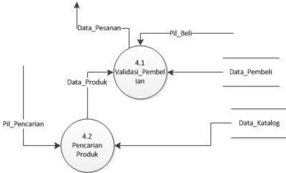
Gambar 6. Diagram Level 2 Proses Pemesanan
