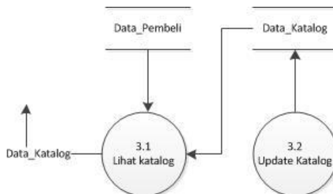
Gambar 5. Diagram Level 2 Proses lihat dan update katalog
