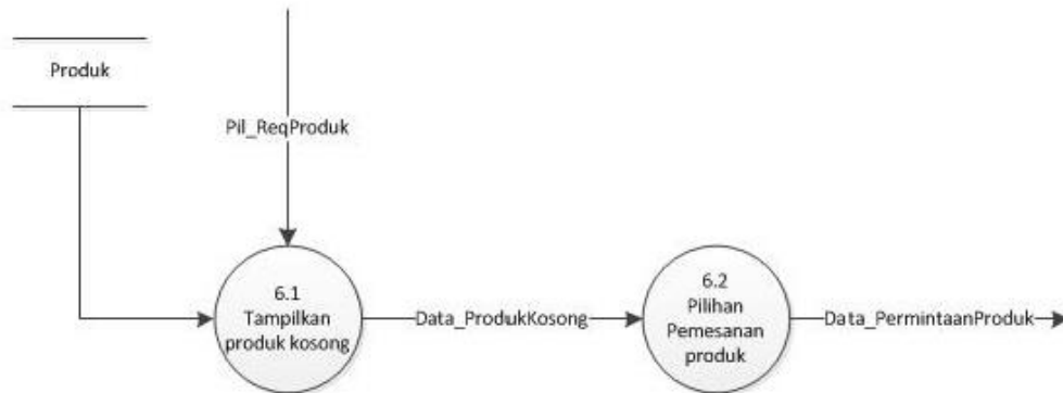
Gambar 8. Diagram Level 2 Proses Permintaan produk
